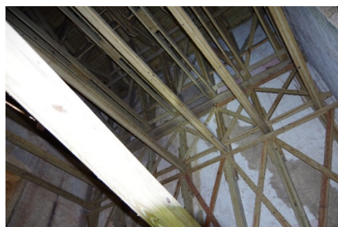
Figure 10: Batterie Coidavid - Étaisement
